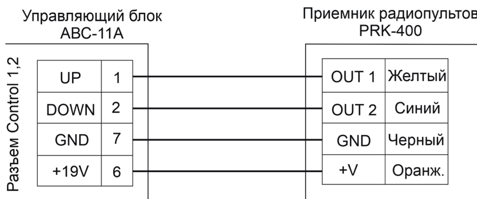
Рисунок 6.6.2.2 Схема подключения приемника радиопультов к управляющему блоку «ABC-11A»
